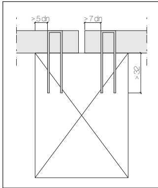
Klammerbefestigung Bepunktung
