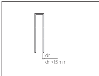
Klammern gemäss DIN 1052-2
